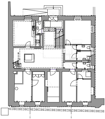
1. Untergeschoss
