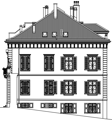
Ostfassade
