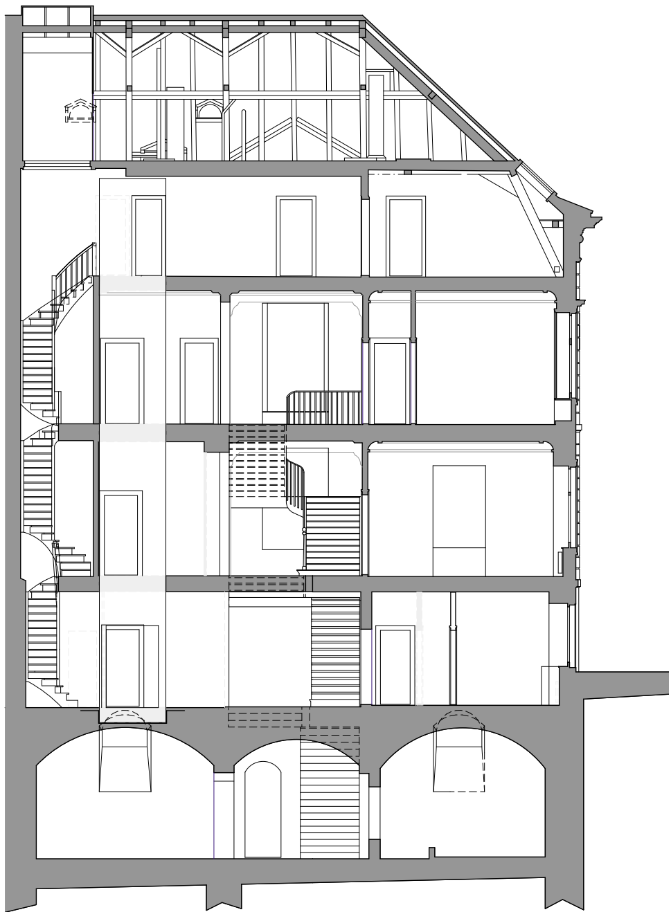
Schnitt A
